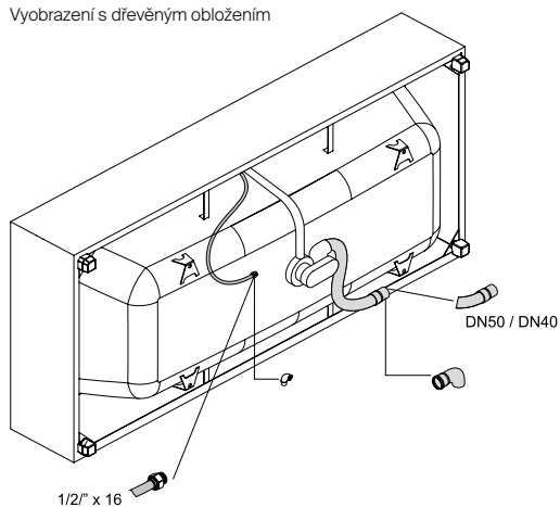
Vyobrazení s dřevěným obložení
