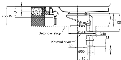
Zobrazení s odtokovou soupravou kolmou - 0,6 l/s výška hladiny 50 mm
