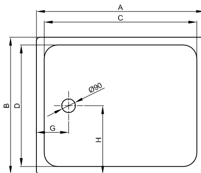
Sprchové vany s ramenem \geq 1000 mm
