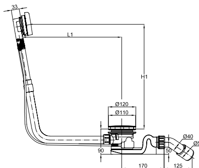
Odtoková soustava plus 5, Ø 90 mm
