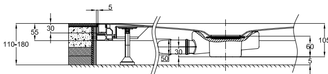
Zobrazení s odtokovou soupravou BetteFloor - 0,85 l/s, výška hladiny 50 mm
