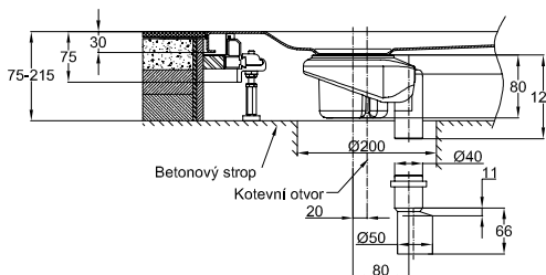
Zobrazení s odtokovou soupravou kolmou - 0,6 l/s, vertikální odtok, výška hladiny 50 mm
