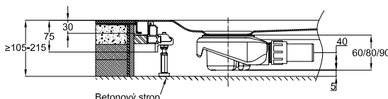
Zobrazení s odtoková souprava - 0,6 l/s, výška hladiny 50 mm
