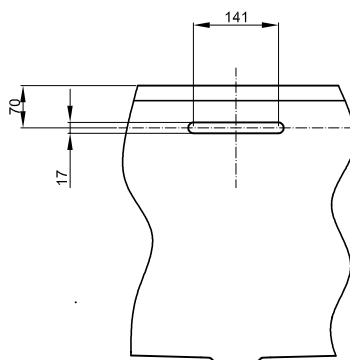
Rozměry výřezu pro přítok
