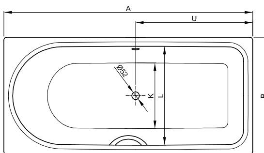
N° 1: strana nohou vpravo, přepad vzadu
