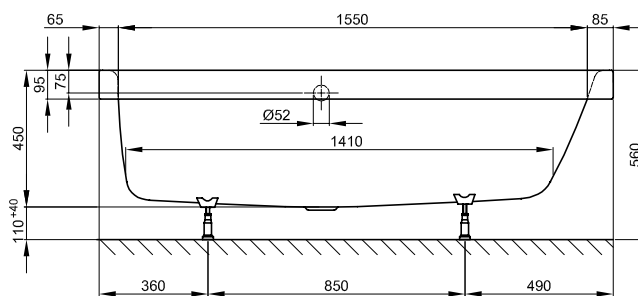
N° 2: strana nohou levá, přepad vpředu
