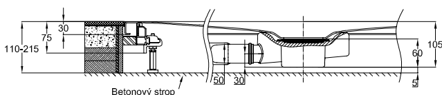
Zobrazení s odtokovou soupravou - 0,85 l/s, boční odtoh, výška hladiny 50 mm
