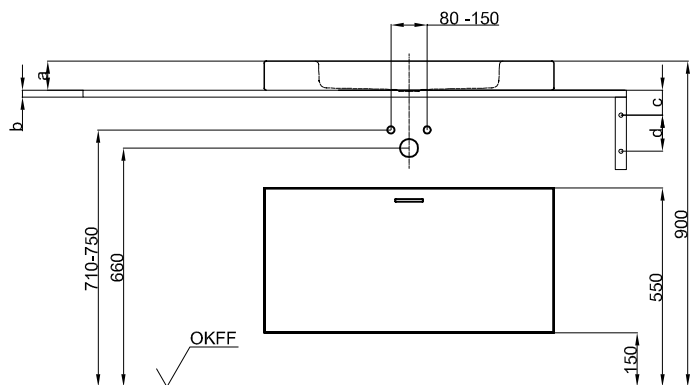
Obr.: Vyobrazení s nábytkem
