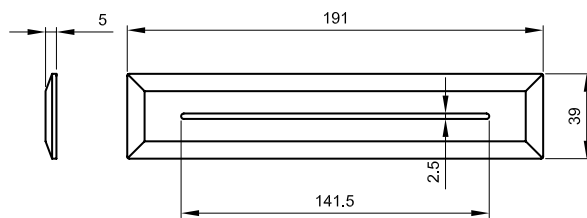
Rozměry výřezu pro přítok
