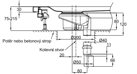
BB573-*, odtoková soustava vertikální 0,6 l/s Obr.: s vertikálním odtokem, výška hladiny 50 mm podle DIN/EN 274
