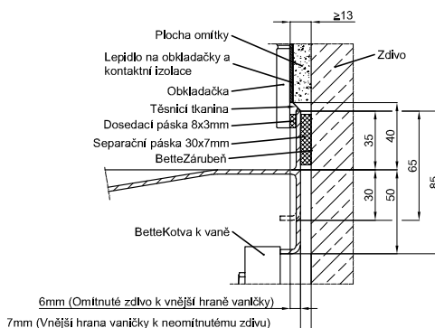
Vestavba na masivní stěnu
