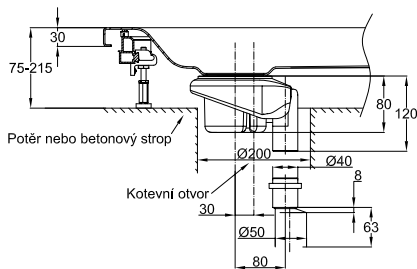
B573-*, odtoková soustava vertikální 0,6 l/s Obr.: s vertikálním odtokem, výška hladiny 50 mm podle DIN/EN 274
