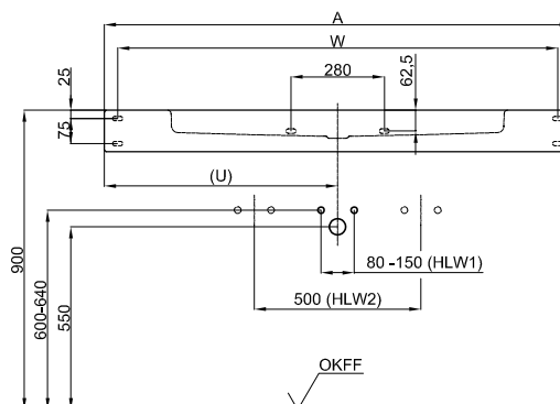
Montážní a přípojovací rozmery:
