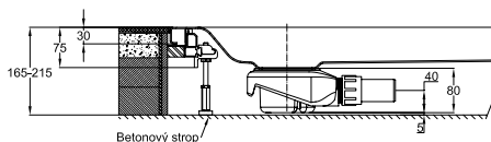
Zobrazení s odtoková souprava - 0,6 l/s, výška hladiny 50 mm
