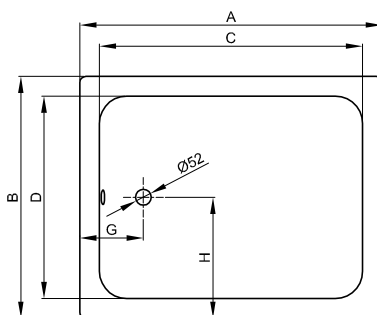
Sprchové vany s ramenem ≥ 1000 mm
