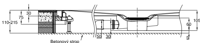
Zobrazení s odtokovou soupravou - 0,85 l/s, boční odtok, výška hladiny 50 mm
