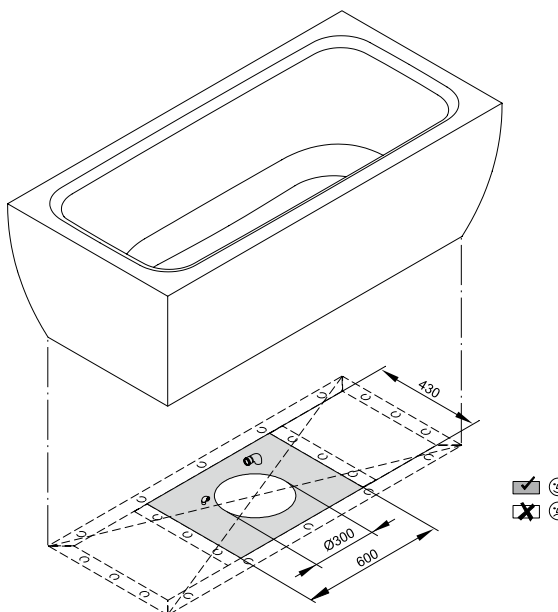
Připojovací rozměry pro odtokovou a přepádivou soustavu
