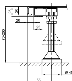
Obr.: Průřez sprchová vanička vč. nosných rámu
