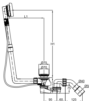
Odtoková soustava plus 5, Ø 52 mm, standard
