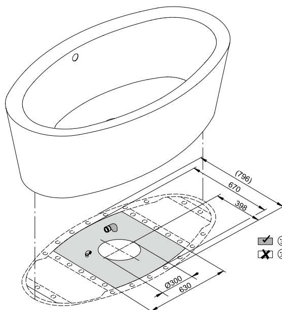
Připojovací rozměry pro odtokovou a přepadovou soustavu
