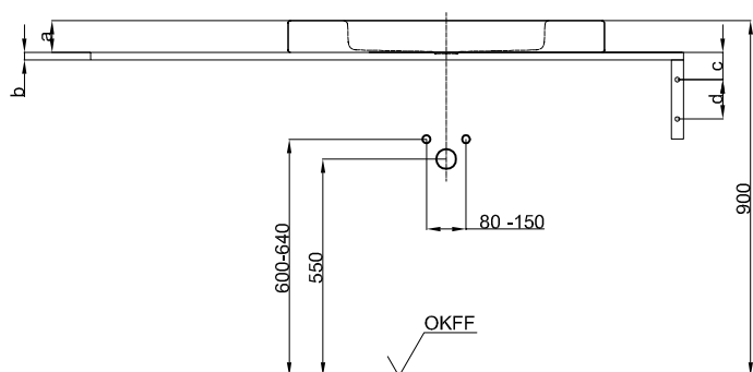
Obr.: Vyobrazení bez nábytku
