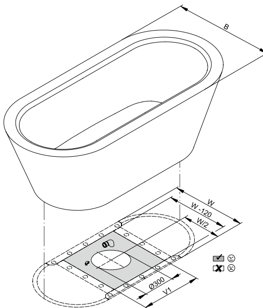
Připojovací rozměry pro odtokovou a přepádivou soustavu
