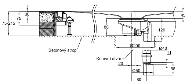
Zobrazení s odtokovou soupravou kolmou - 0,6 l/s, vertikální odtok, výška hladiny 50 mm
