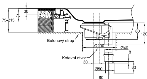
Zobrazení s odtokovou soupravou kolmou - 0,6 l/s výška hladiny 50 mm
