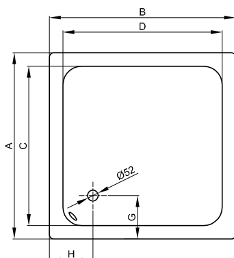
Sprchové vany s ramenem < 900 mm
