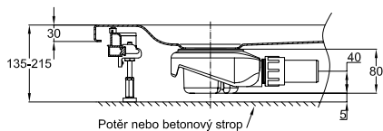
B572-*, odtoková soustava 0,6 l/s Obr.: s bočním odtokem, výška hladiny 50 mm podle DIN/EN 274
