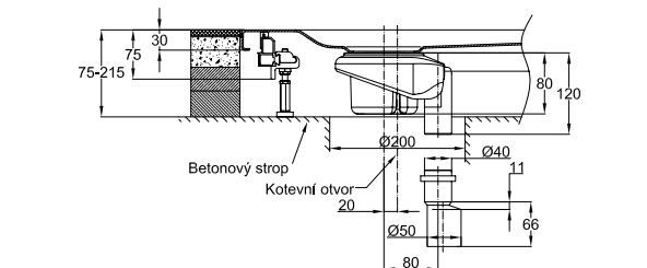
B573-*, odtoková soustava vertikální 0,6 l/s Obr.: s vertikálním odtokem, výška hladiny 50 mm podle DIN/EN 274
