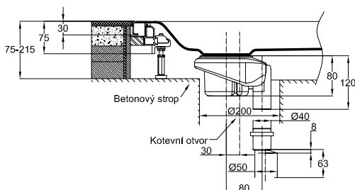
Zobrazení s odtokovou soupravou kolmou - 0,6 l/s výška hladiny 50 mm
