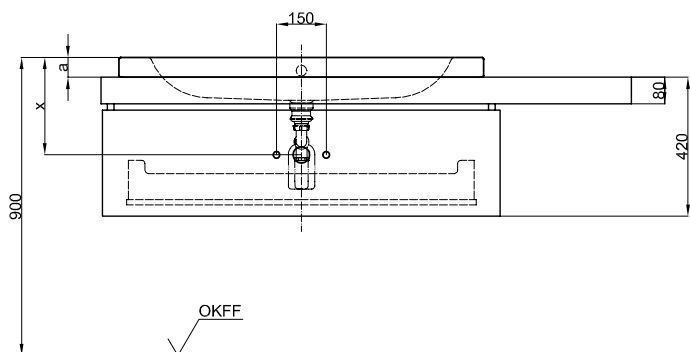
Obr.: Vyobrazení s BetteRoom Modul pro umístění pod desku
