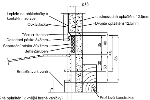
Vestavba na odlehčenou stěnu
