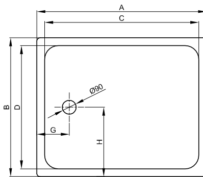
Sprchové vany s ramenem \geq 1000 mm
