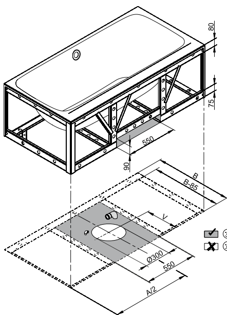
Připojovací rozměry pro odtokovou a přepádovou soustavu
