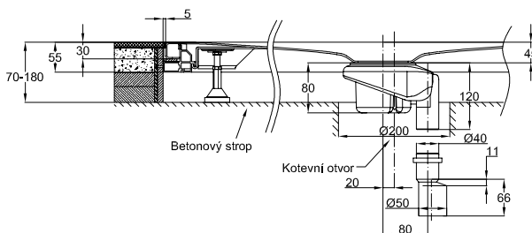
Vertikální odtoh - 0,6 l/s, Ø 90 mm, výška hladiny 50 mm
