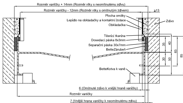
Vestavba na masivní stěnu
